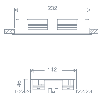
TOLEDO encastré
